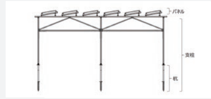
▲ソーラーパネルをのせる「藤棚式」架台。高さが2~4mほどで、丸山さんの架台高は約3m、その上部に50cmほどの隙間をあけてパネルを設置。パネルの下はトラクターなどの農業機械が使えるよう、支柱の間隔も3~4mと広い。
